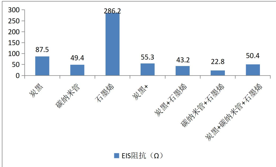
图表 29：不同导电剂的阻抗对比
